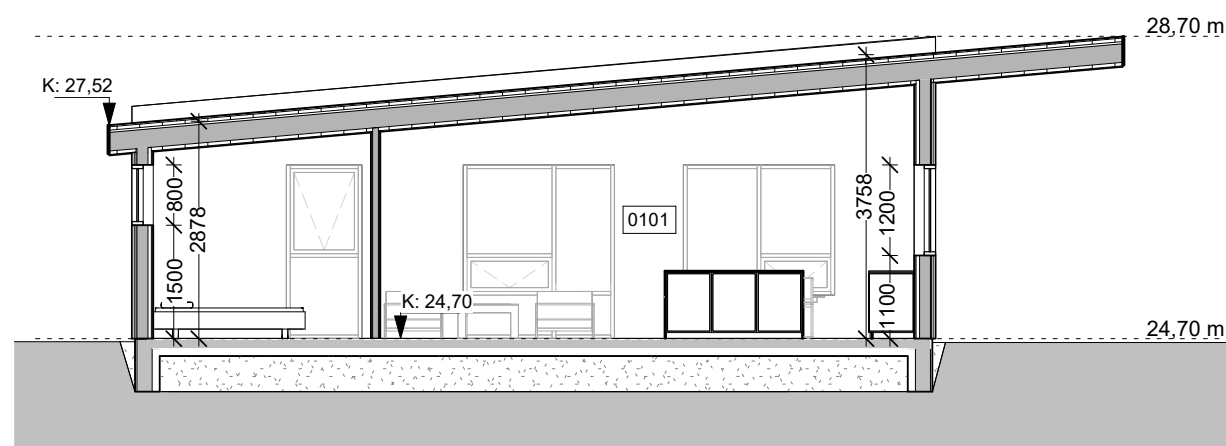
Snið B-B 1 : 100
