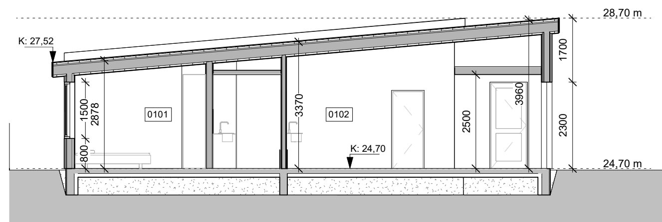
Snið A-A 1 : 100
