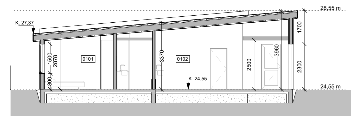
Snið A-A 1 : 100
