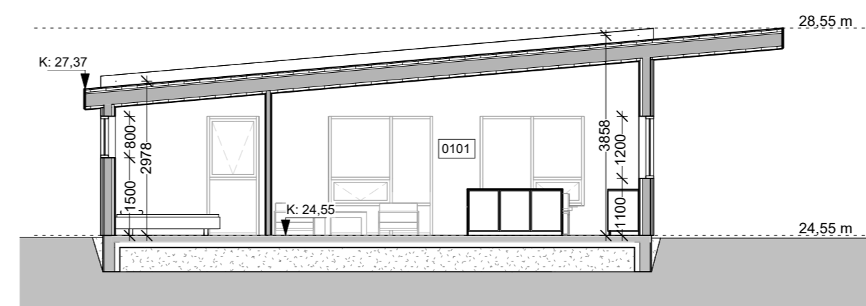
Snið B-B 1 : 100
